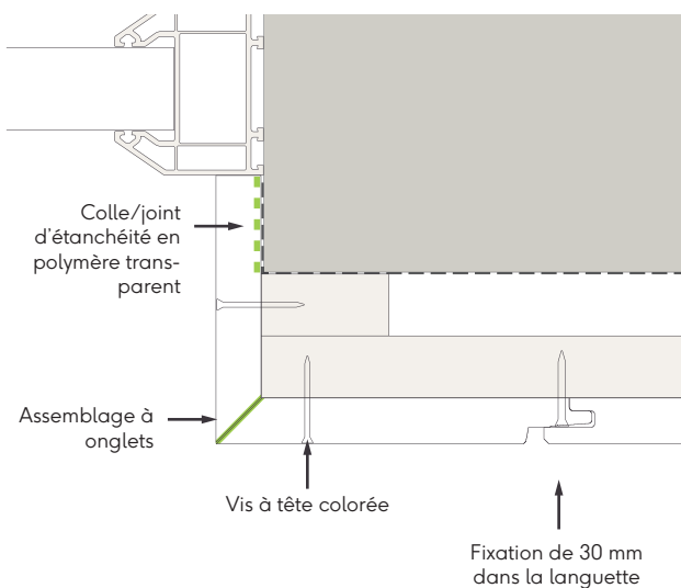
Fig. 13 - Montant de la fenêtre/porte avec joint biseauté
