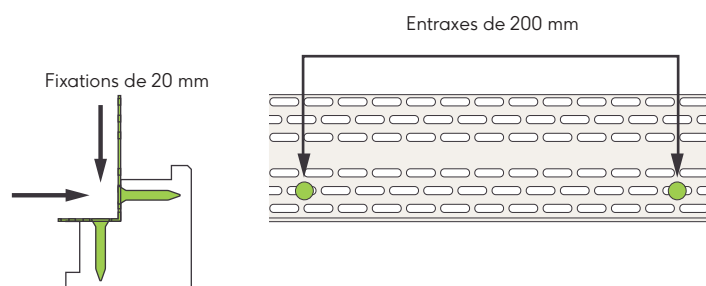
Fig. 6 - Utilisation de grilles anti-nuisibles perforées sur les profils d'angle
