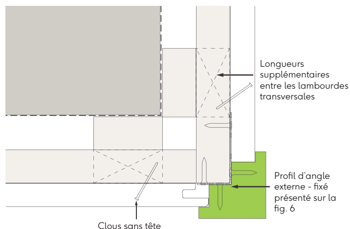
Fig. 16 - Détail du coin externe - clous sans tête
