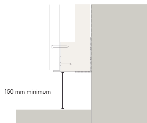
Fig. 4 - Détail de l'installation au-dessus du niveau du sol
