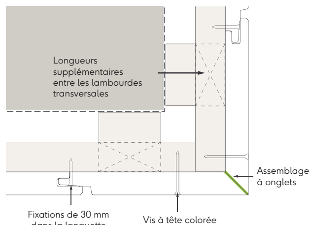
Fig. 10 - Détail du coin biseauté externe
