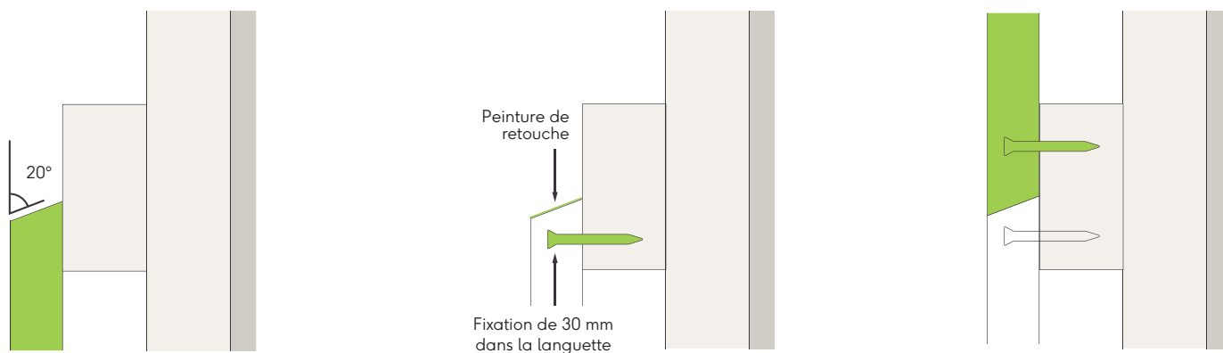
Figure 20 : détails de l'assemblage des lames
