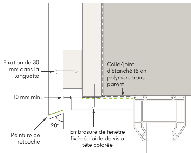
Fig. 15 - Embrasure de fenêtre/porte avec biseau
