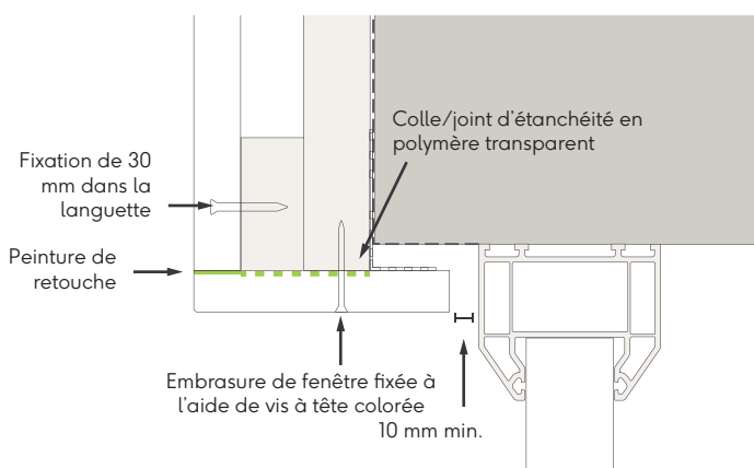
Fig. 12 - Chambranle de fenêtre/porte avec lames pour embrasure
