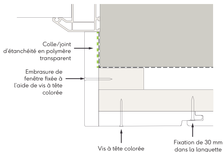
Fig. 11 - Montant de fenêtre/porte avec lame pour embrasure
