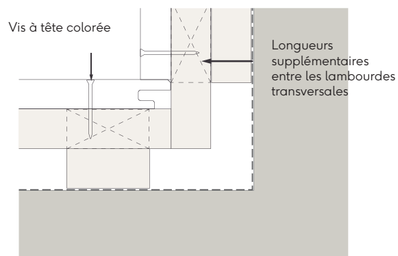
Fig. 9 - Détail d'assemblage bout à bout interne
