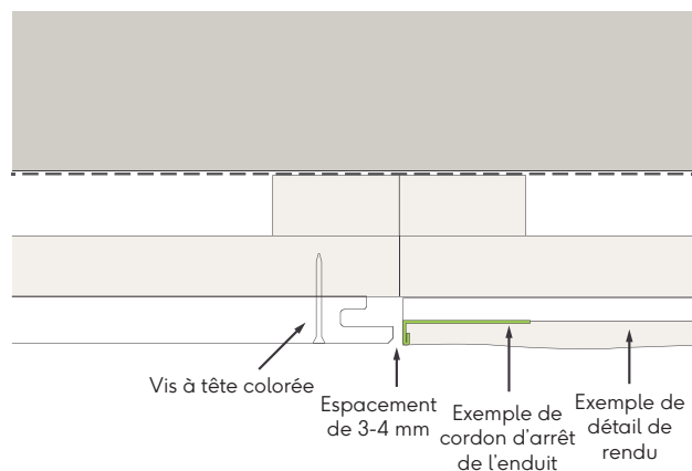
Fig. 21 - Profil d'angle jusqu'à l'enduit
