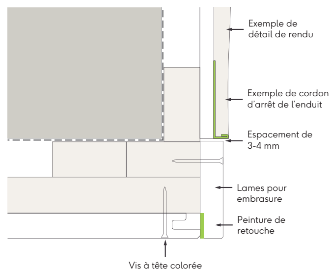
Fig. 22 - Profil d'angle jusqu'à l'enduit sur le coin externe
