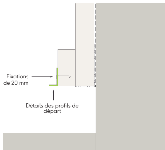
Figure 18b : détails des profils de départ
