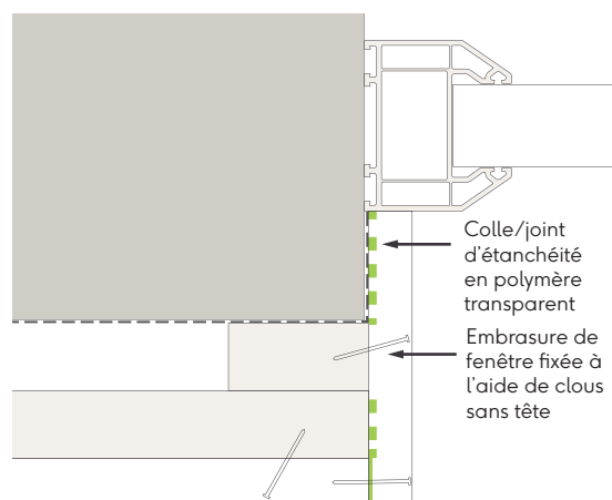
Fig. 17 - Montant de fenêtre/porte avec lame pour embrasure - clous sans tête
