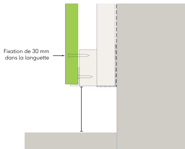
Fig. 19 - Installation de la première lame
