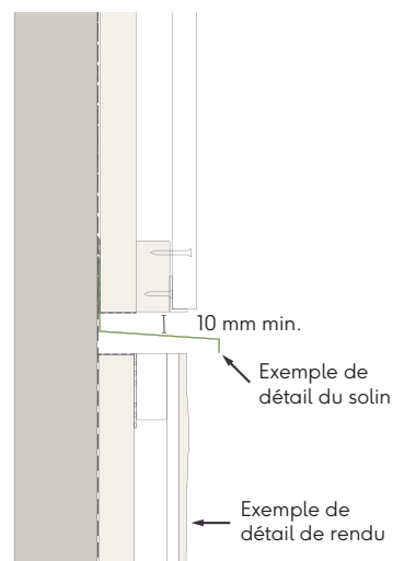
Fig. 23 - Installation du bardage au-dessus de l'enduit
