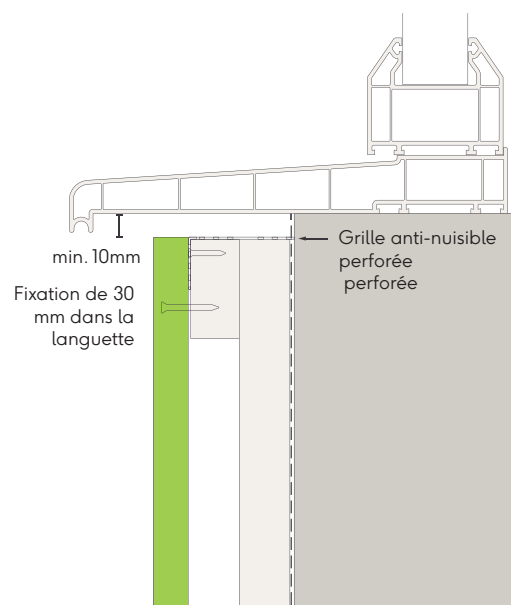
Fig. 3 - Détail du rebord de fenêtre/seuil de porte
