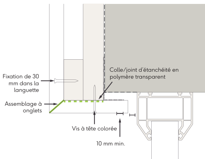
Fig. 14 - Chambranle de fenêtre/porte avec joint biseauté
