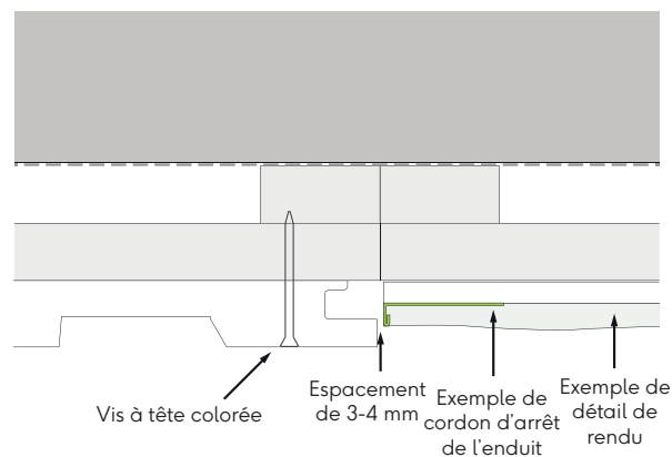
Fig. 19 - Profil d'angle jusqu'à l'enduit
