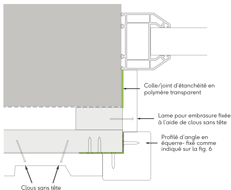
Fig. 15 - Détail de la jonction avec un rebord de fenêtre/ porte - Clous sans tête
