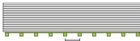
Assurez-vous que les lames reposent sur une surface plane ou des supports espacés de 400 mm maximum
