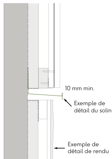
Fig. 21 - Installation du bardage au-dessus de l'enduit
