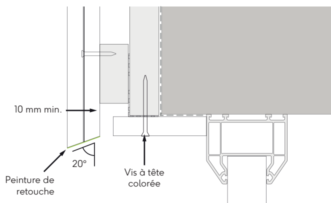
Fig. 14 - Chambranle de fenêtre/ porte avec biseau
