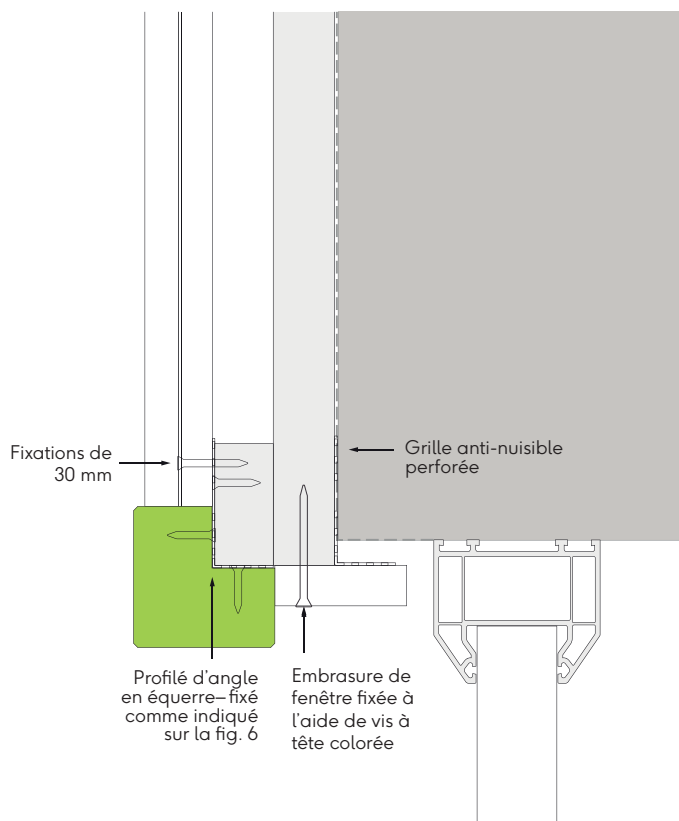
Fig. 12 - Chambranle de fenêtre / porte avec profilé d'angle
