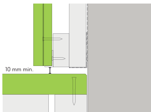
Fig. 5 - Détail de l'installation au-dessus du platelage
