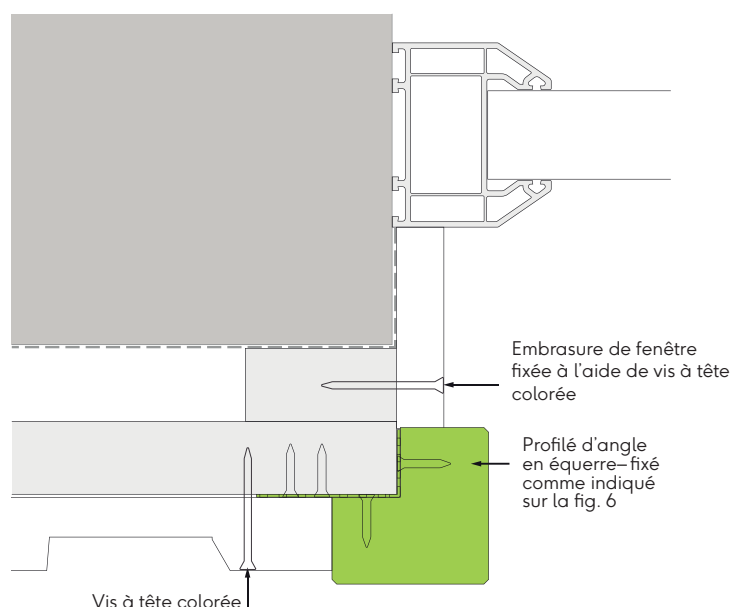
Fig. 11 - Montant de fenêtre / porte avec profil de rive
