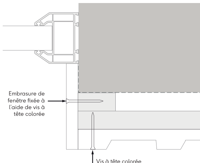
Fig. 13 - Montant de fenêtre/ porte avec lames pour embrasure
