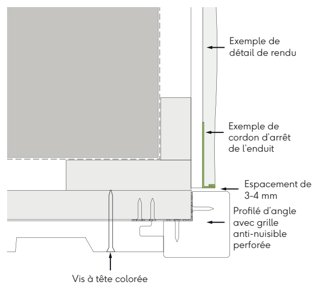
Fig. 20 - Profil d'angle jusqu'à l'enduit sur l'angle externe
