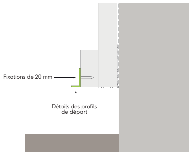
Figure 16b : détails des profils de départ
