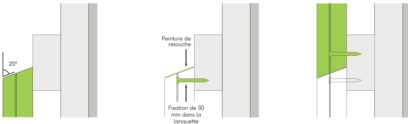
Figure 18 : détails de l'assemblage des lames
