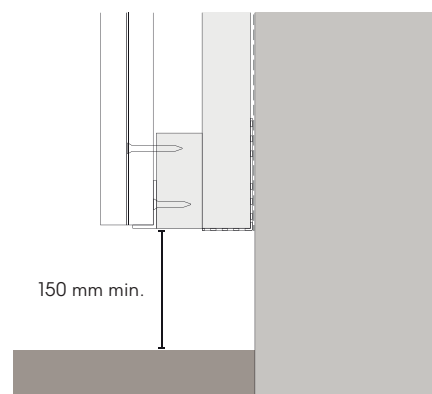
Fig. 4 - Détail de l'installation au-dessus du niveau du sol
