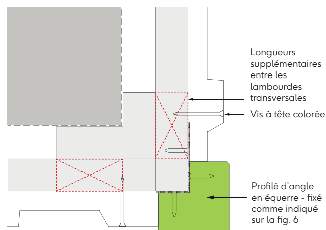
Fig. 8 - Détail de l'angle externe
