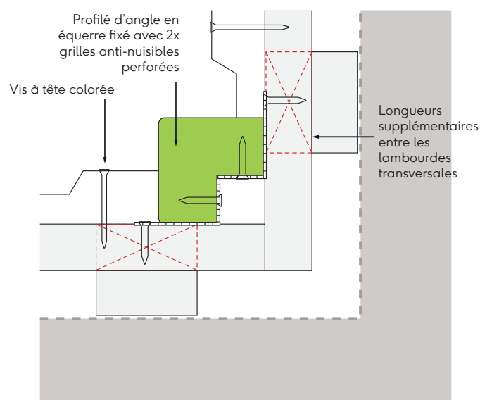
Fig. 7 - Détail de l'angle interne
