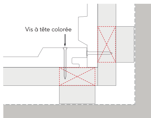
Fig. 9 - Détail de l'assemblage bout à bout interne
