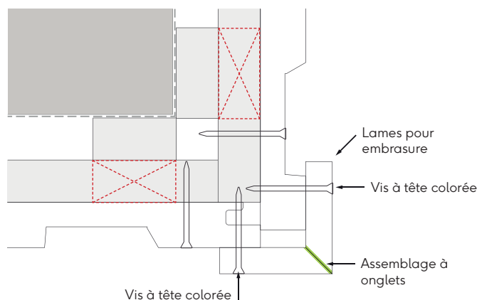
Fig. 10 - Détail de l'angle biseauté externe
