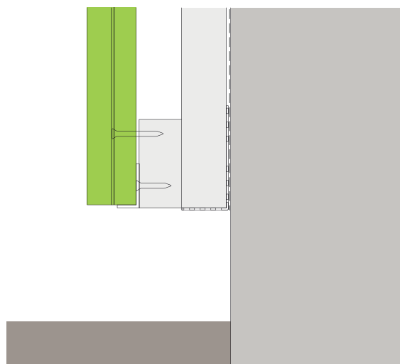
Fig. 17 - Installation de la première lame
