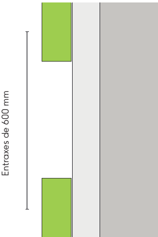
Fig. 2 - Entraxe des lambourdes
