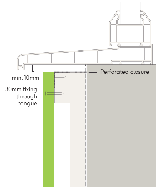
Fig. 3 - Window / door sill detail
