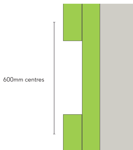
Fig. 2 - Batten centres
