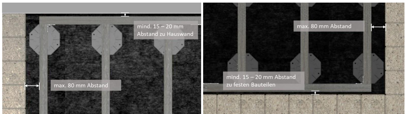
Bild 11. Durch die Größe der Bodenplatte von den Verstellfüßen ca. 200 mm, wird der Abstand der Unterkonstruktion zu der Stein- Umrandung definiert und sollte max. 80 mm betragen. Zur Hauswand und festen Bauteilen (z.B. Steinumrandung) 15 – 20 mm
