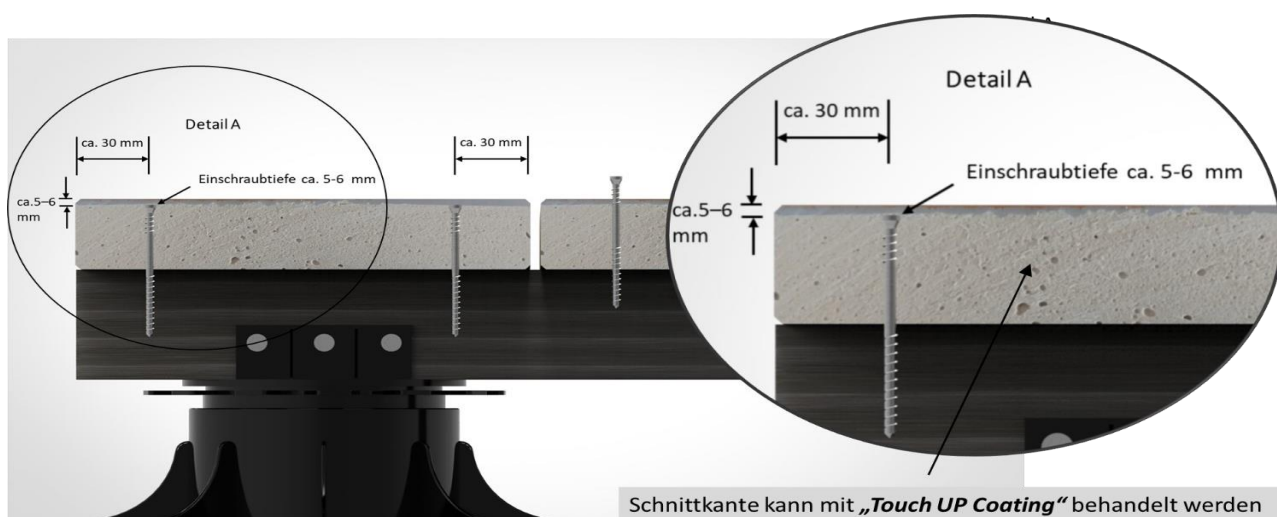
Bild 14. Die Durafix Schrauben® müssen ca. 5 - 6 mm tief eingedreht werden und zur Längskante der Dielen ca. 30 mm Abstand haben.
