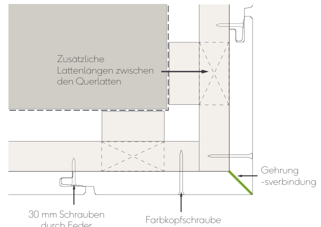
Abb. 10 - Details der auf Gehrung geschnittenen Außenecke
