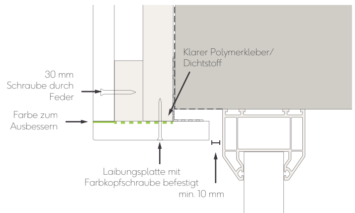
Abb. 12 - Fenster-/Türsturz mit Laibungsplatte
