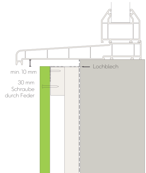
Abb. 3 - Detail Fenster/Türschwelle
