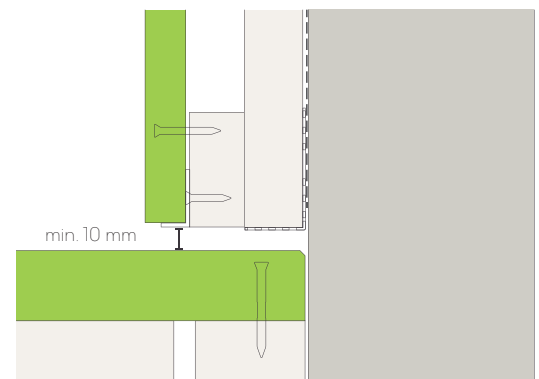
Abb. 5 - Einbaudetails über Terrassendiele
