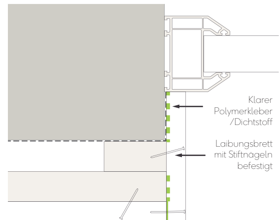
Abb. 17 - Fenster-/Türpfosten mit Laibungsplatte - Stiftnägel
