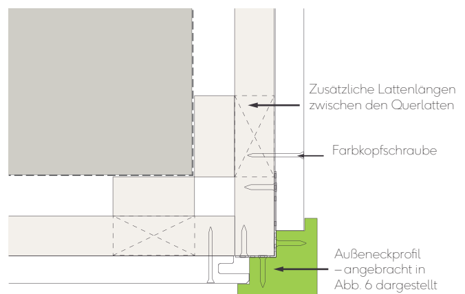
Abb. 8 - Details der Außenecke
