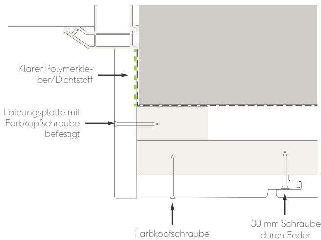
Abb. 11 - Fenster-/Türpfosten mit Laibungsplatte
