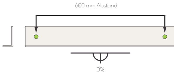
Abb. 18a - Anfangszierleiste
