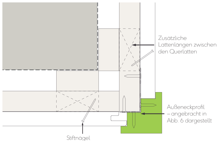
Abb. 16 - Details der Außenecke - Stiftnägel
