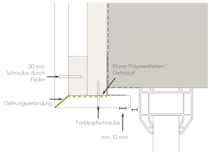
Abb. 14 - Fenster-/Türsturz mit Gehrungsverbindung
