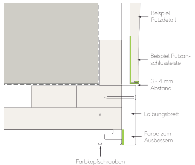
Abb. 22 - Eckprofil stoßt an der Außenecke an den Putz an
