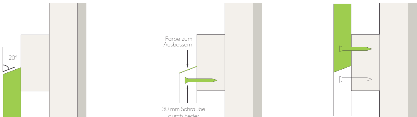
Abb. 20 - Detail zum Verbinden von Paneelen
