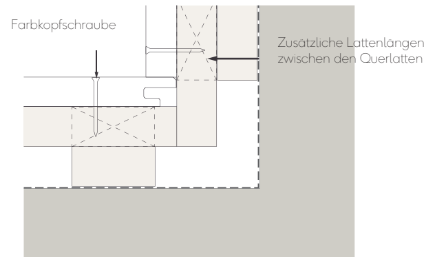
Abb. 9 - Detail der Innenstoßecke
