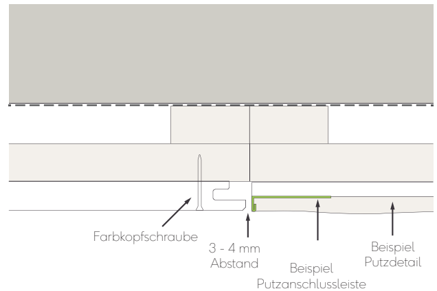
Abb. 21 - Eckprofil stoßt an den Putz an
