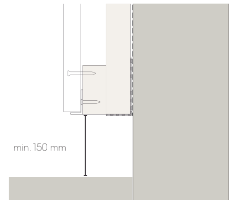
Abb. 4 - Einbaudetail über Bodenhöhe
