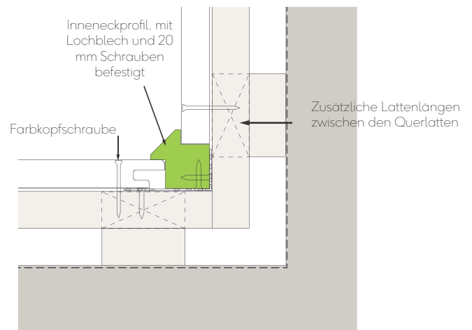
Abb. 7 - Details der Innenecke
