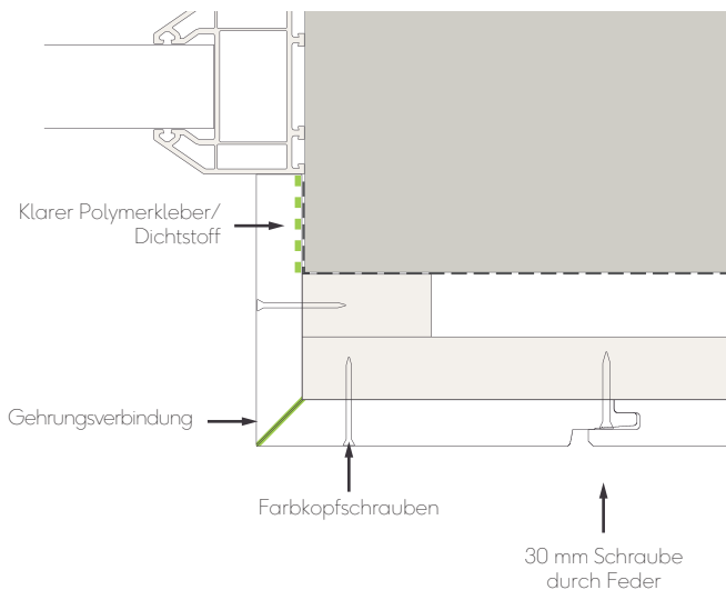
Abb. 13 - Fenster-/Türpfosten mit Gehrungsverbindung
