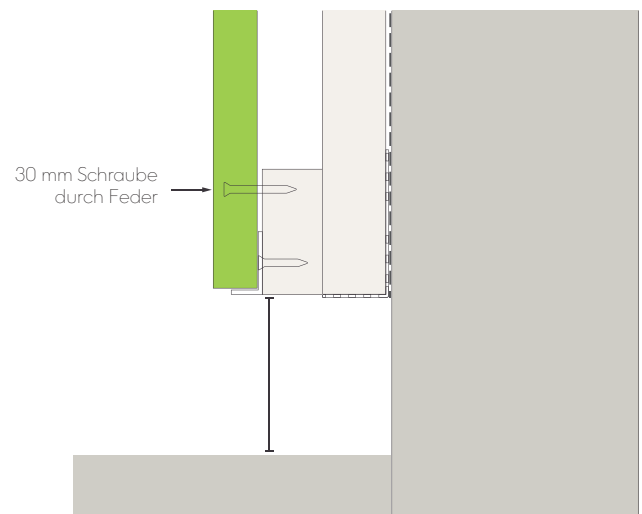
Abb. 19 - Erste Paneelmontage
