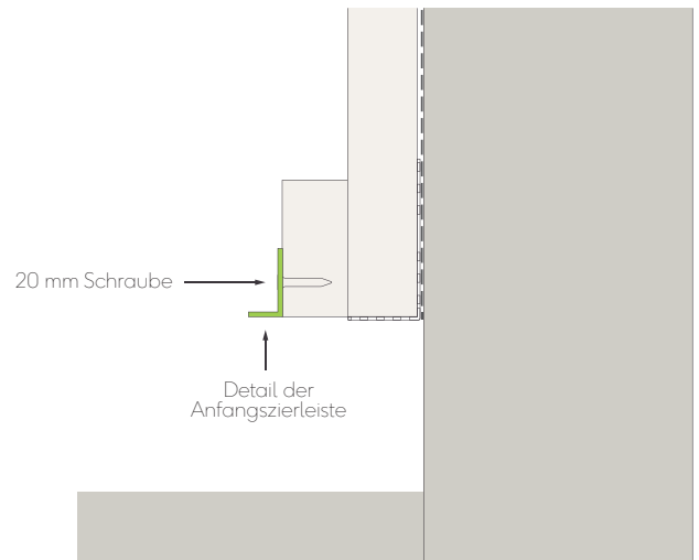
Abb. 18b - Detail der Anfangszierleiste
